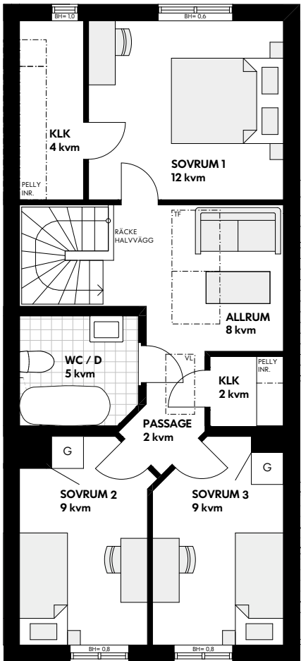
Övre plan
