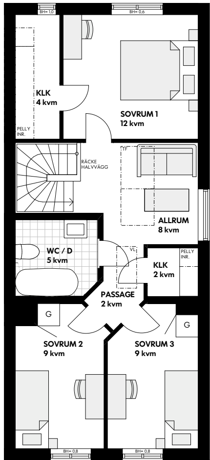
Övre plan
