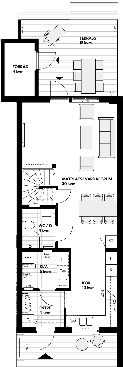
Entréplan
