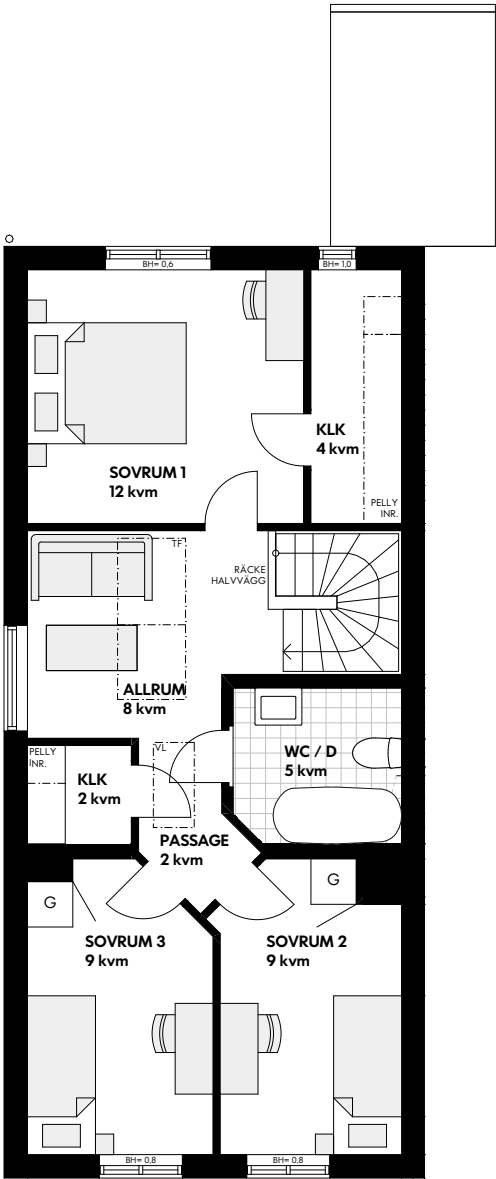
Övre plan
