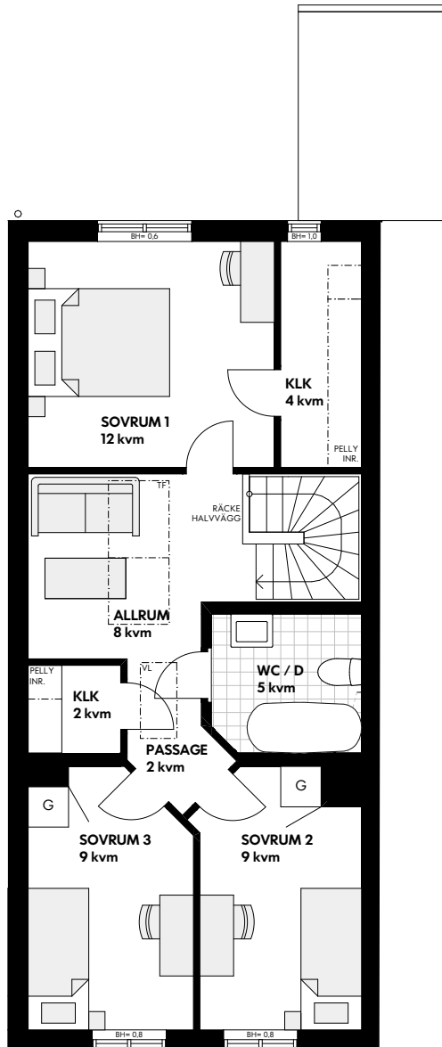
Övre plan
