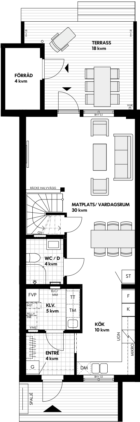
Entréplan
