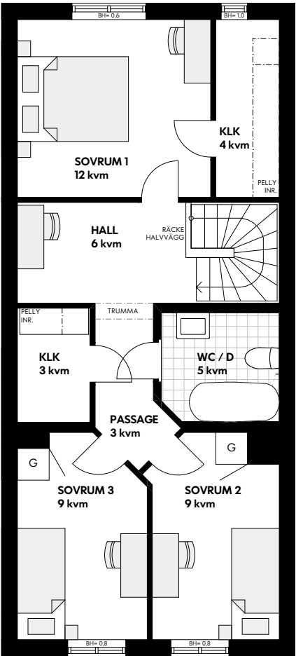
Övre plan
