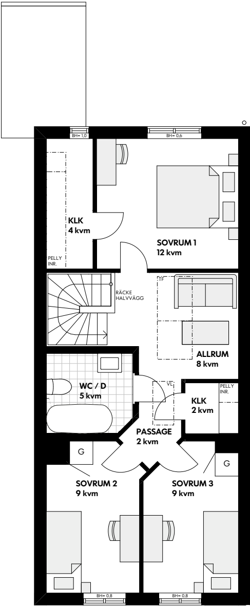
Övre plan
